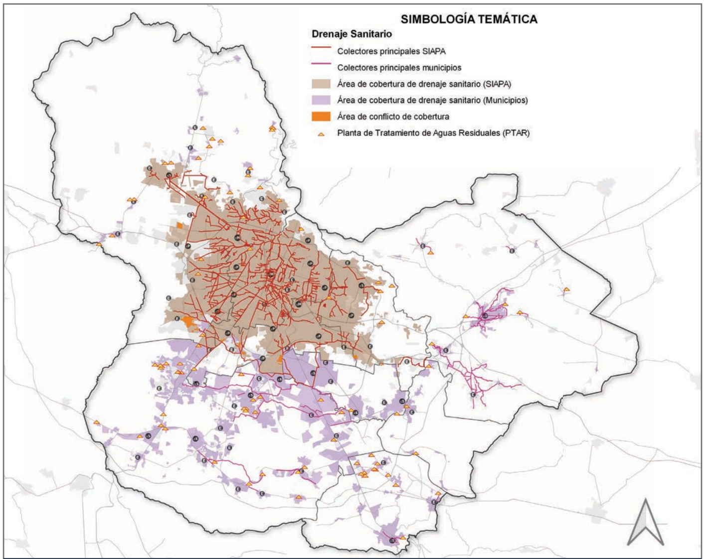
Cobertura de drenaje sanitario Elaboración propia con datos del Inventario de Infraestructura Estratégica de Imeplan.
