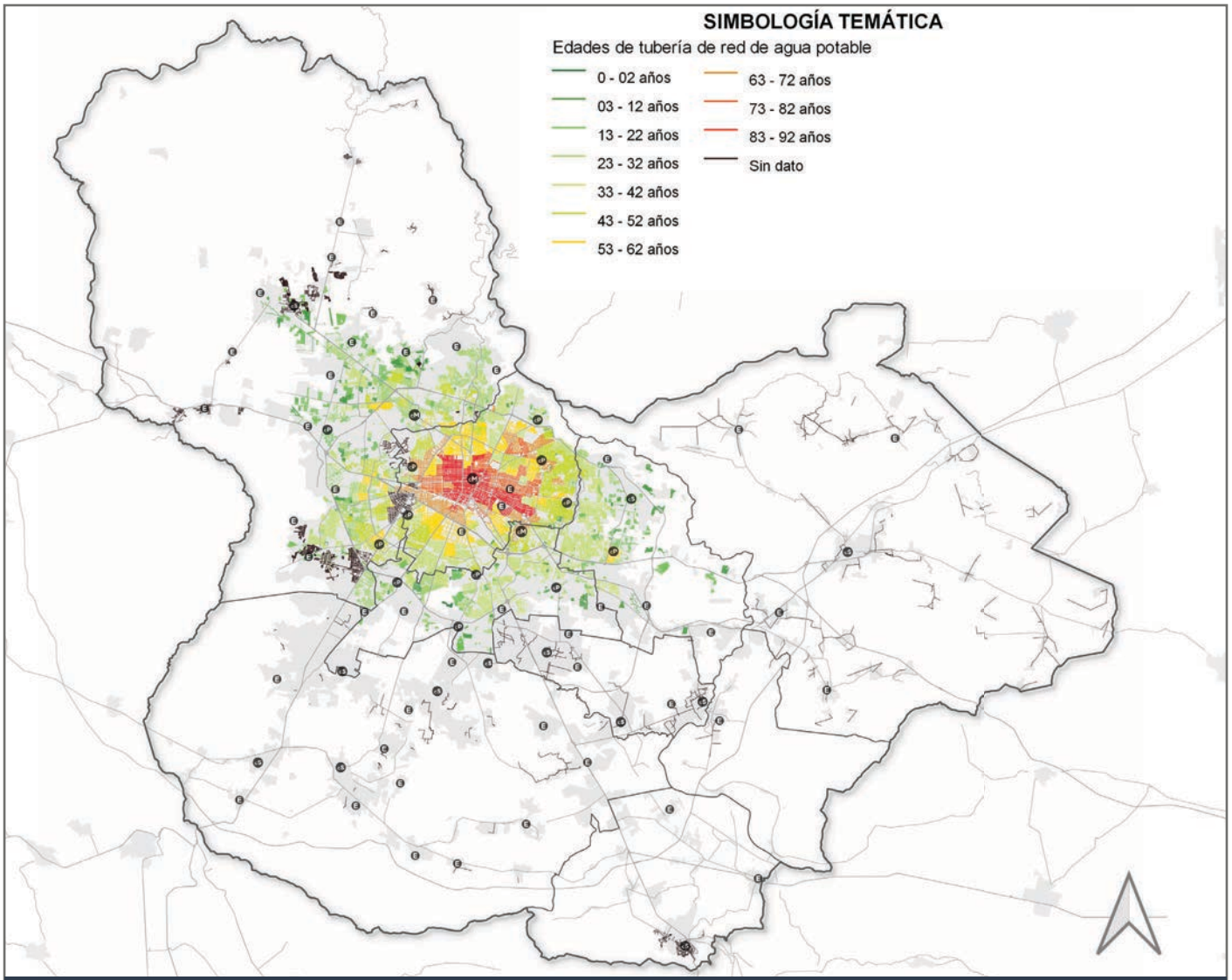
Edades de tubería de la red de agua potable Elaboración propia con datos del Inventario de Infraestructura Estratégica de Imeplan.
