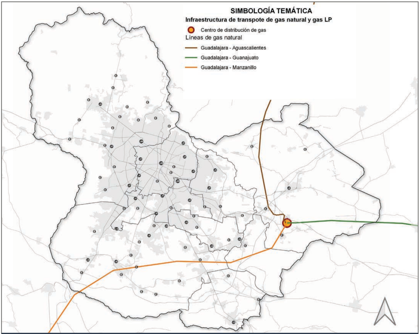
Infraestructura de transporte de gas natural y gas LP Elaboración propia con datos del Mapa Jalisco del Gobierno del Estado de Jalisco (2023).
