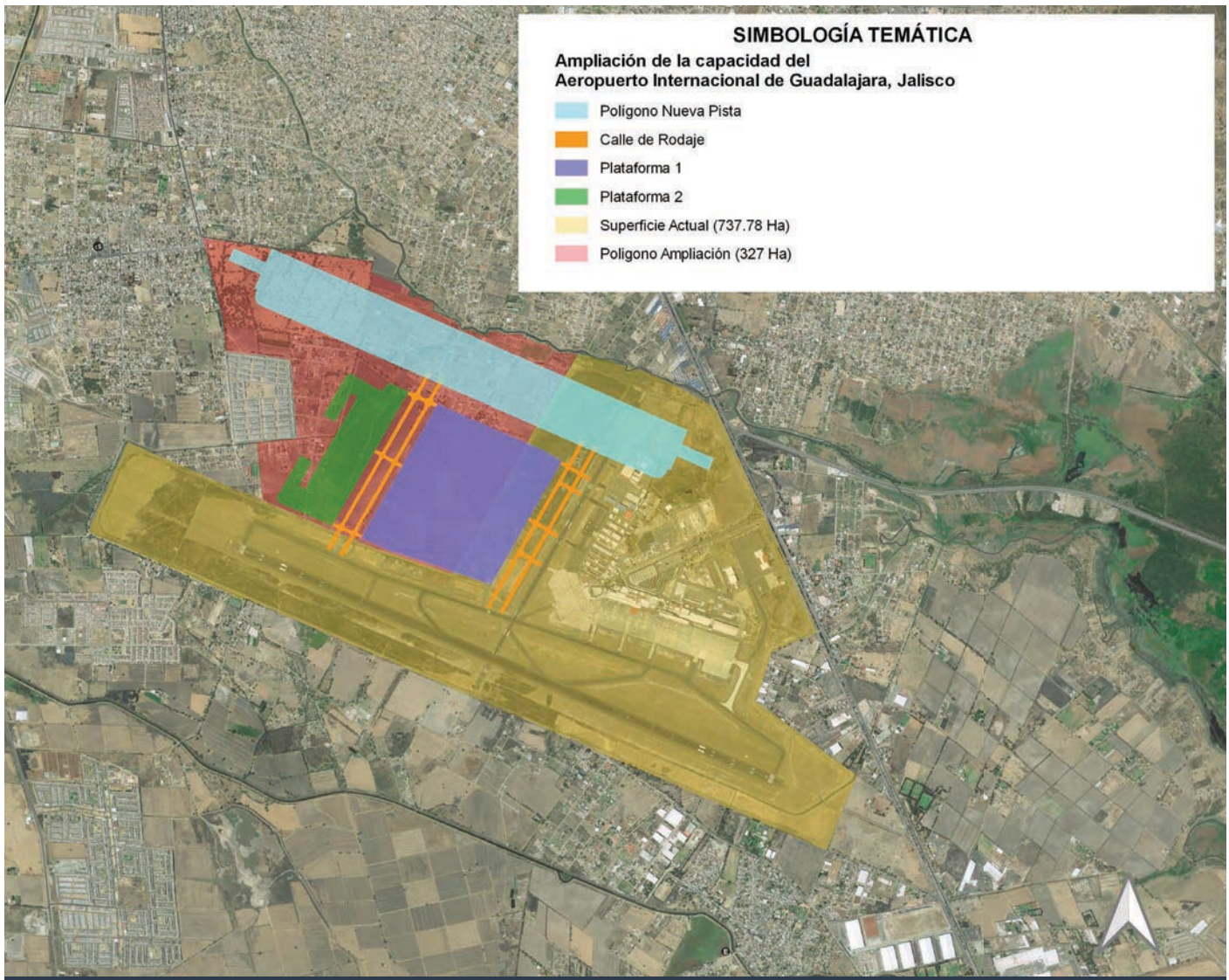
Ubicación de la superficie adicional para la ampliación del Aeropuerto Internacional de Guadalajara. Elaboración propia con datos de SICT (n.d).
