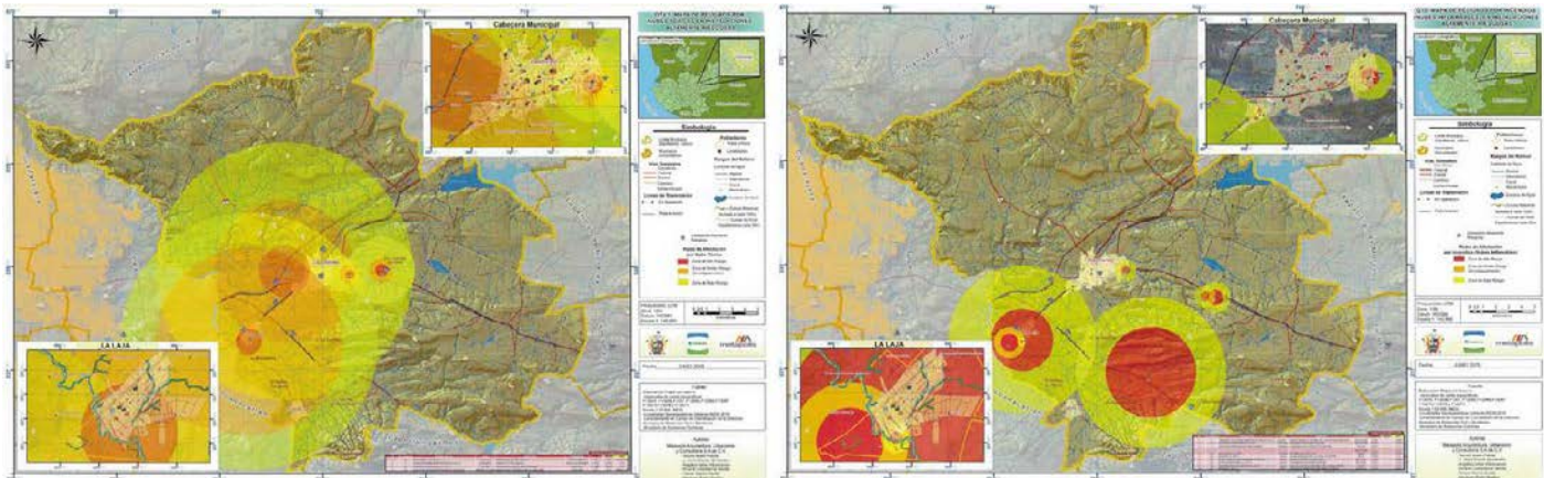
Ejemplos de radios de alto riesgo por nube tóxica (izquierda) y explosión (derecha) en el municipio de Zapotlanejo Atlas Integral de peligros y Riesgos del municipio de Zapotlanejo del Gobierno de Zapotlanejo (2015).
